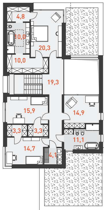
RZUT PODDASZA 131,7 m 2
