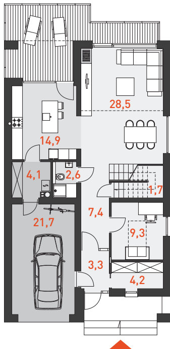
RZUT PARTERU 71,9 m 2
