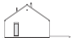
ELEWACJA OGRODOWA
