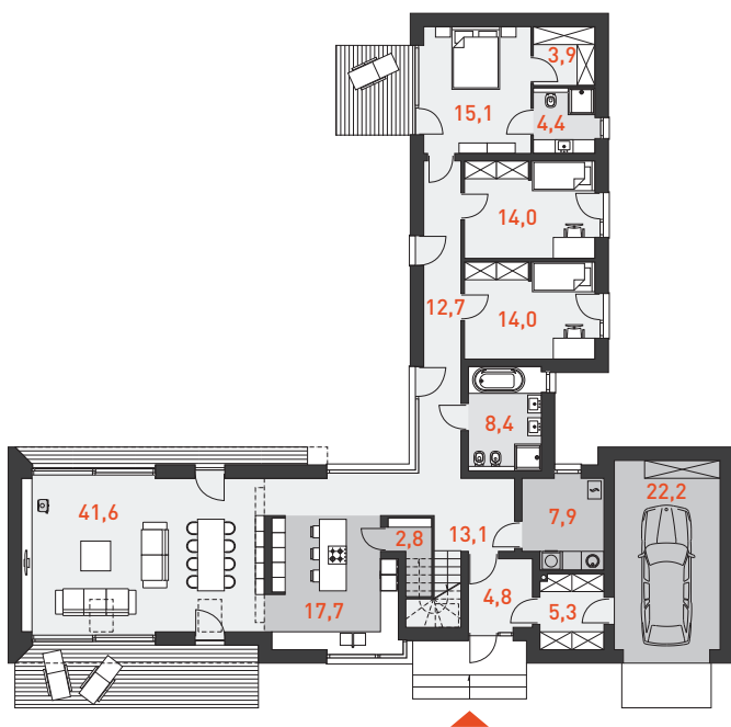
RZUT PARTERU 157,8 m 2
