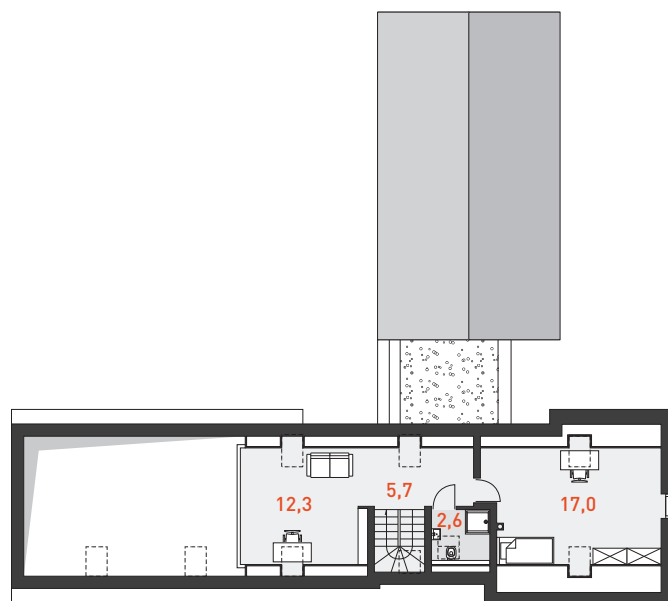
RZUT PODDASZA 37,6 m 2
