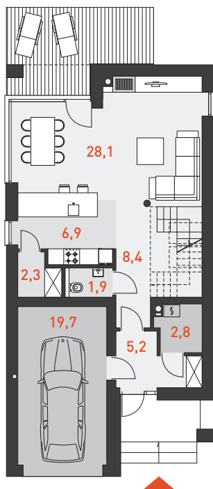
RZUT PARTERU 52,8 m 2
