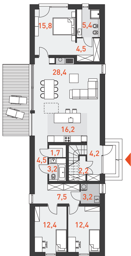
RZUT PARTERU 118,4 m 2
