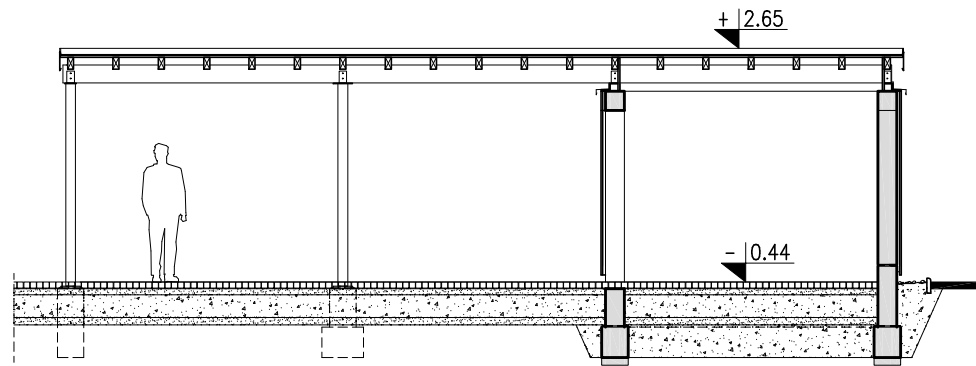
PRZEKRÓJ B-B
