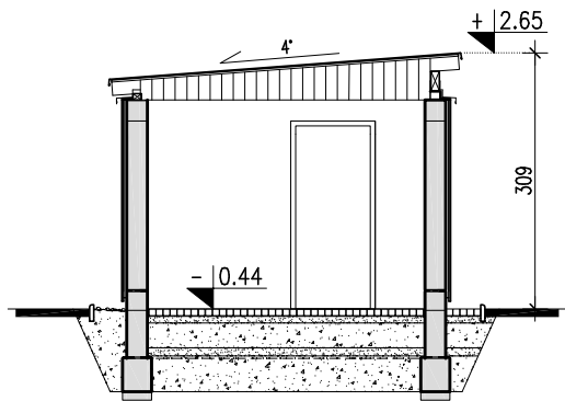
PRZEKRÓJ A-A
