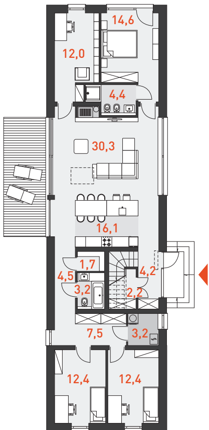
RZUT PARTERU 125,5 m 2
