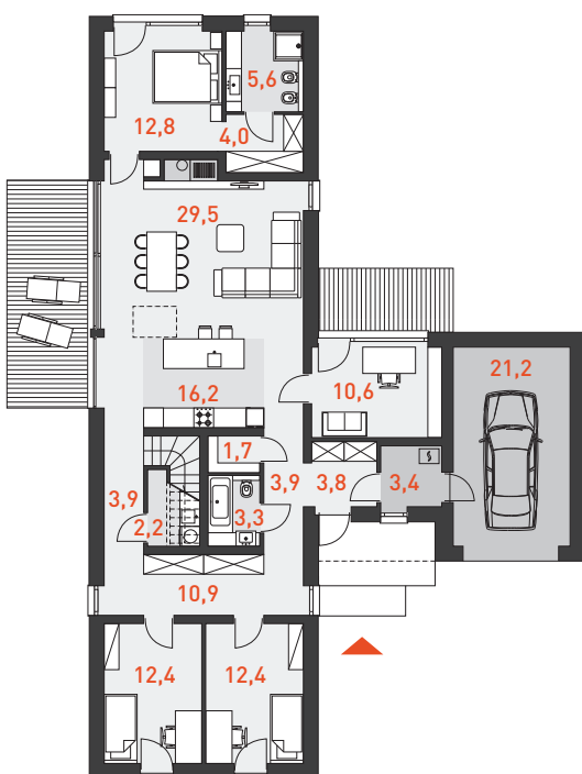
RZUT PARTERU 133,2 m 2
