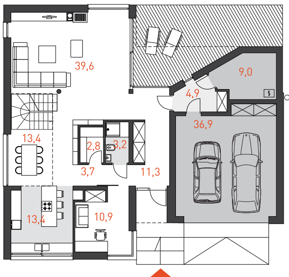
RZUT PARTERU 148,7 m 2
