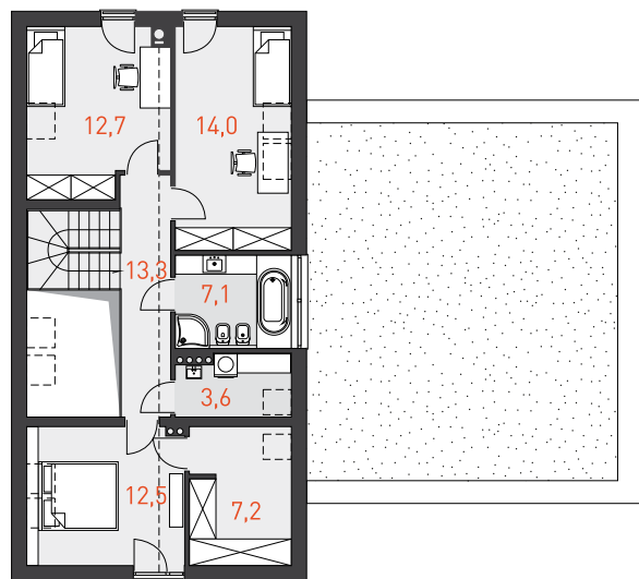
RZUT PODDASZA 69 m 2
