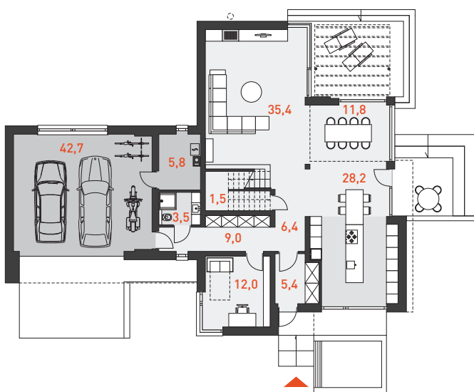
RZUT PARTERU 113,2 m 2
