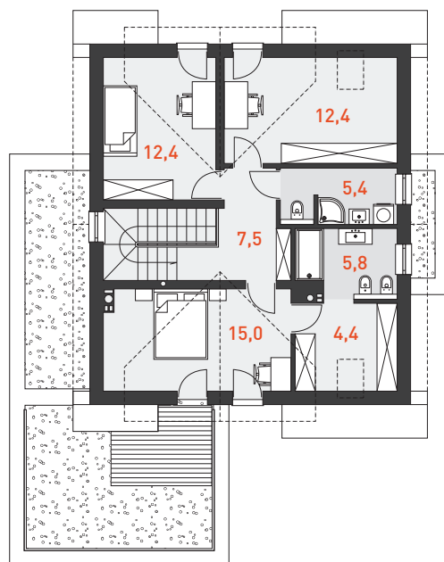
RZUT PODDASZA 63,0 m 2
