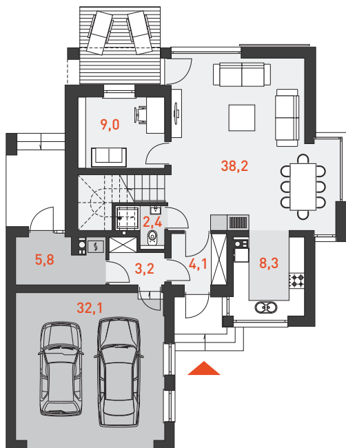
RZUT PARTERU 65,2 m 2
