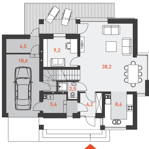
RZUT PARTERU 67,0 m 2
