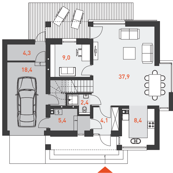
RZUT PARTERU 71,4 m 2
