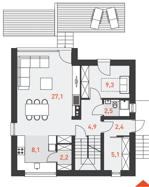
RZUT PARTERU 61,6 m 2
