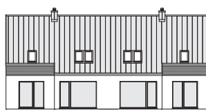
ELEWACJA OGRODOWA
