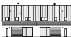
ELEWACJA FRONTOWA
