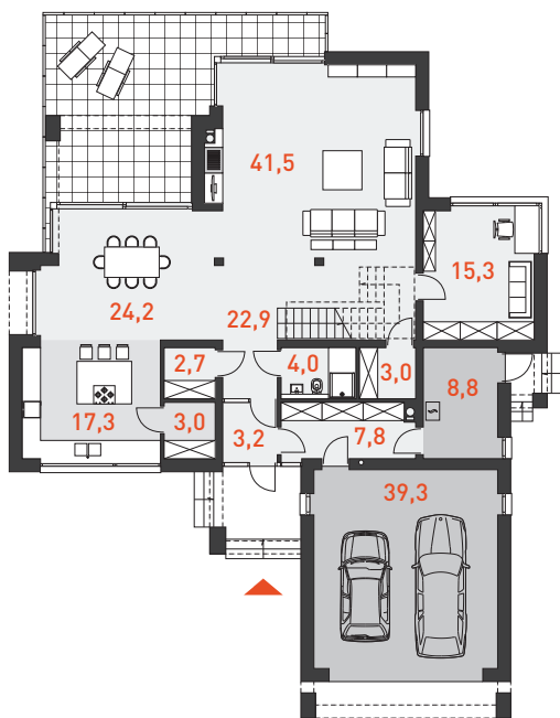
RZUT PARTERU 144,8 m 2
