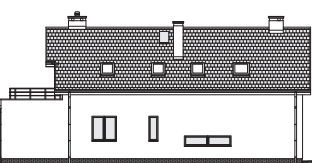
ELEWACJA OGRODOWA
