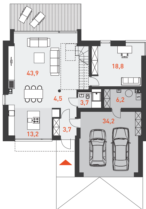
RZUT PARTERU 87,8 m 2
