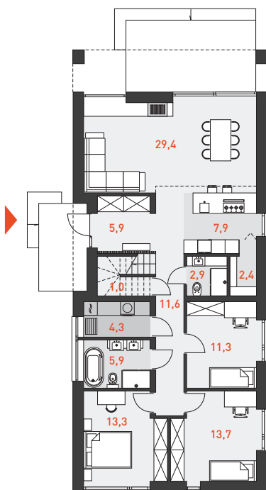
RZUT PARTERU 105,3 m 2
