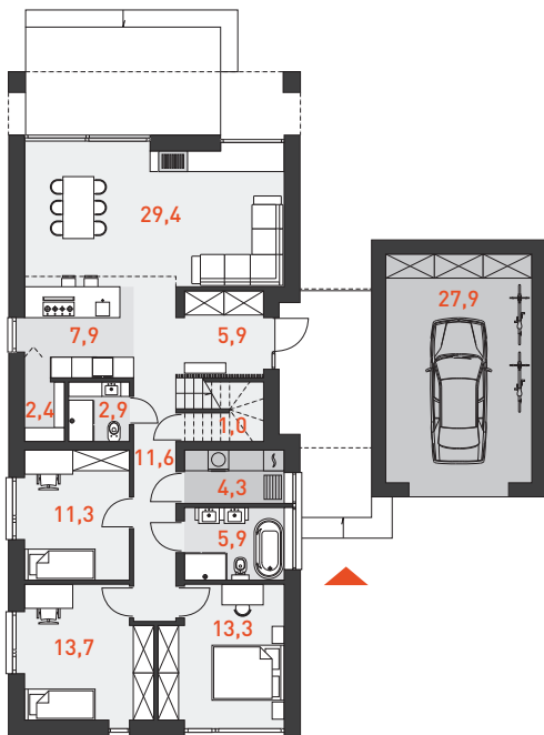
RZUT PARTERU 105,3 m 2
