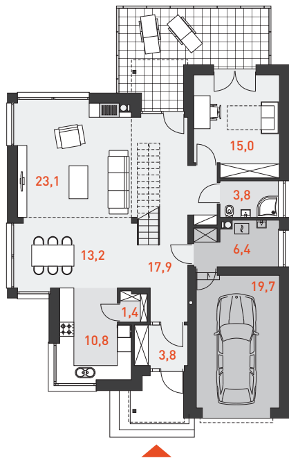
RZUT PARTERU 88,9 m 2
