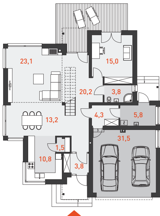
RZUT PARTERU 95,7 m 2
