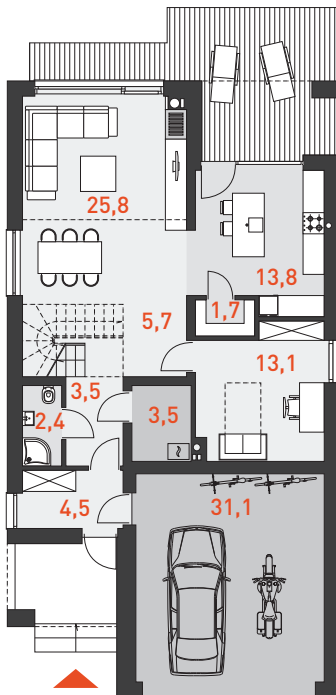
RZUT PARTERU 70,5 m 2
