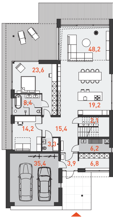
RZUT PARTERU 145,1 m 2
