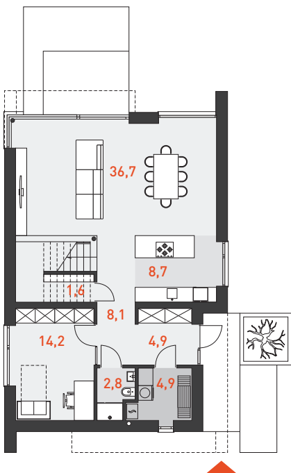
RZUT PARTERU 77,0 m 2
