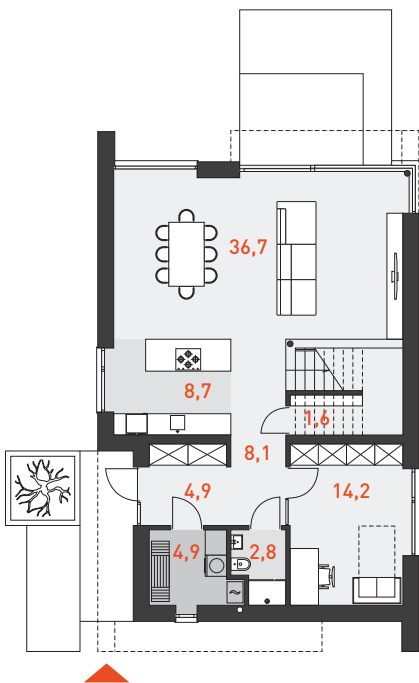
RZUT PARTERU 77,5 m 2
