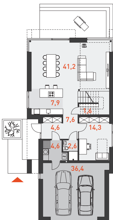
RZUT PARTERU 79,8 m 2
