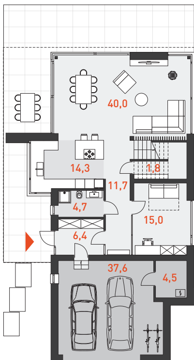
RZUT PARTERU 136,0 m 2
