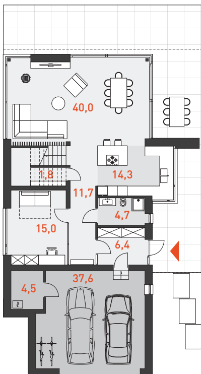
RZUT PARTERU 136,0 m 2
