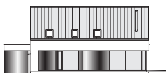
ELEWACJA OGRODOWA
