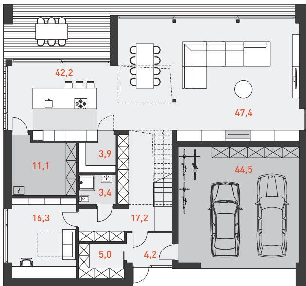
RZUT PARTERU 139,6 m 2
