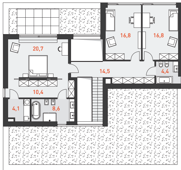
RZUT PIĘTRA 96,3 m 2
