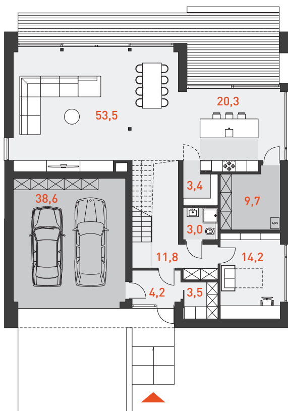
RZUT PARTERU 113,9 m 2
