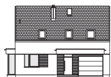
ELEWACJA FRONTOWA
