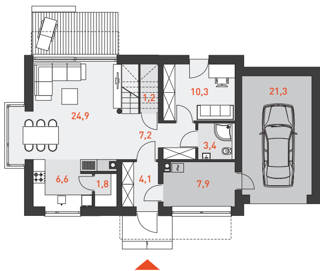
RZUT PARTERU 59,5 m 2
