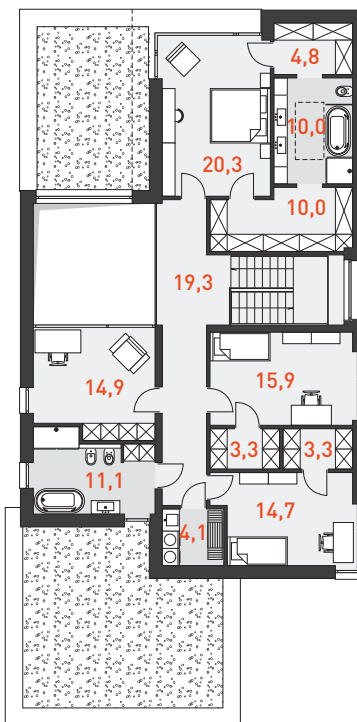
RZUT PODDASZA 131,7 m 2
