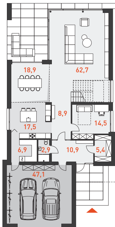
RZUT PARTERU 141,7 m 2
