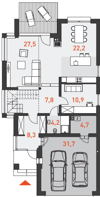
RZUT PARTERU 80,9 m 2
