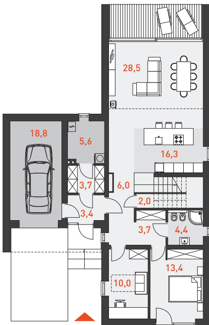
RZUT PARTERU 91,4 m 2
