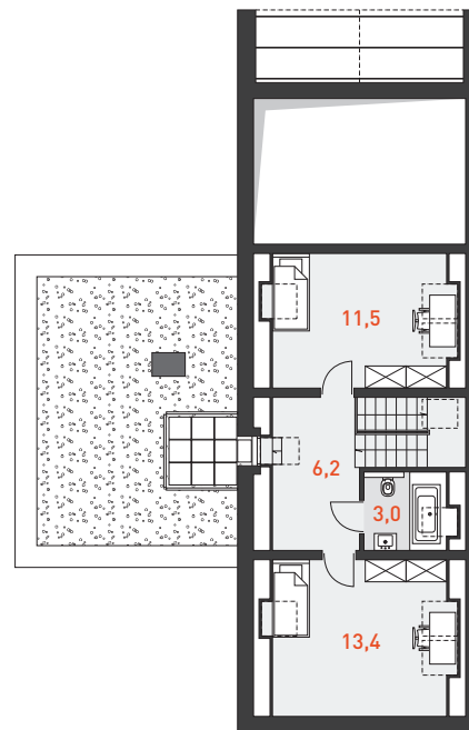
RZUT PODDASZA 34,1 m 2
